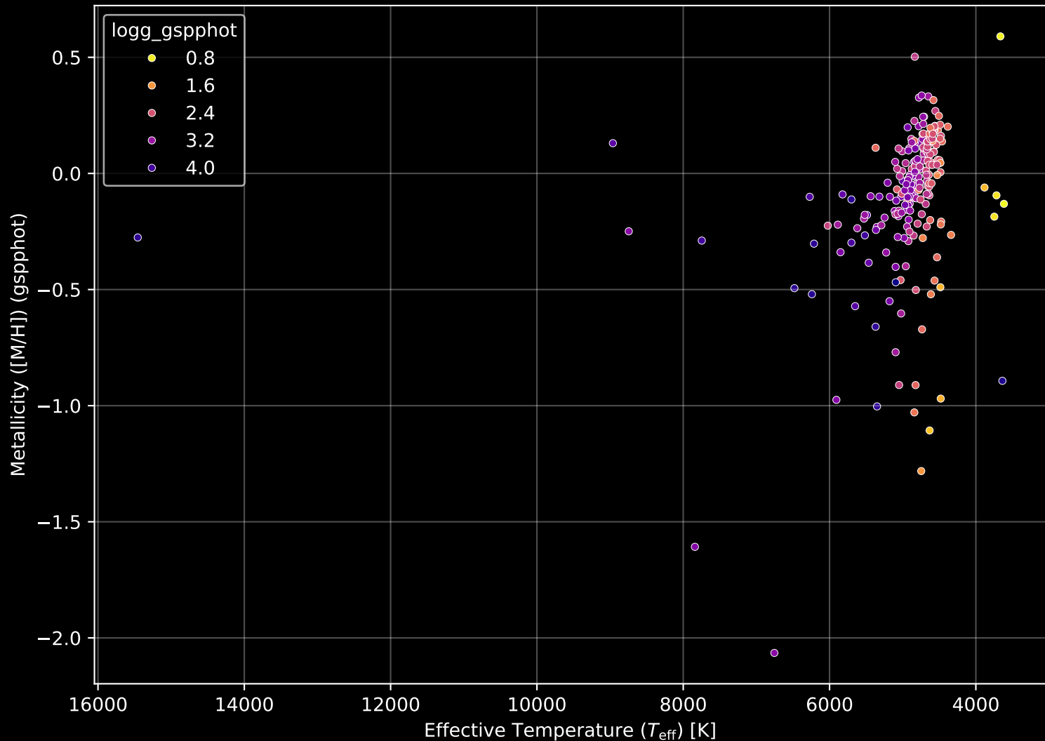
APOGEE DR17 Field: [N6388] Stellar Population Parameters (n= 237)
